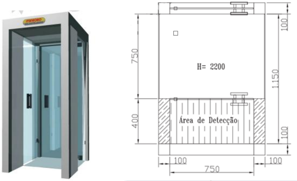
PEDM modelo 2 da tabela acima
