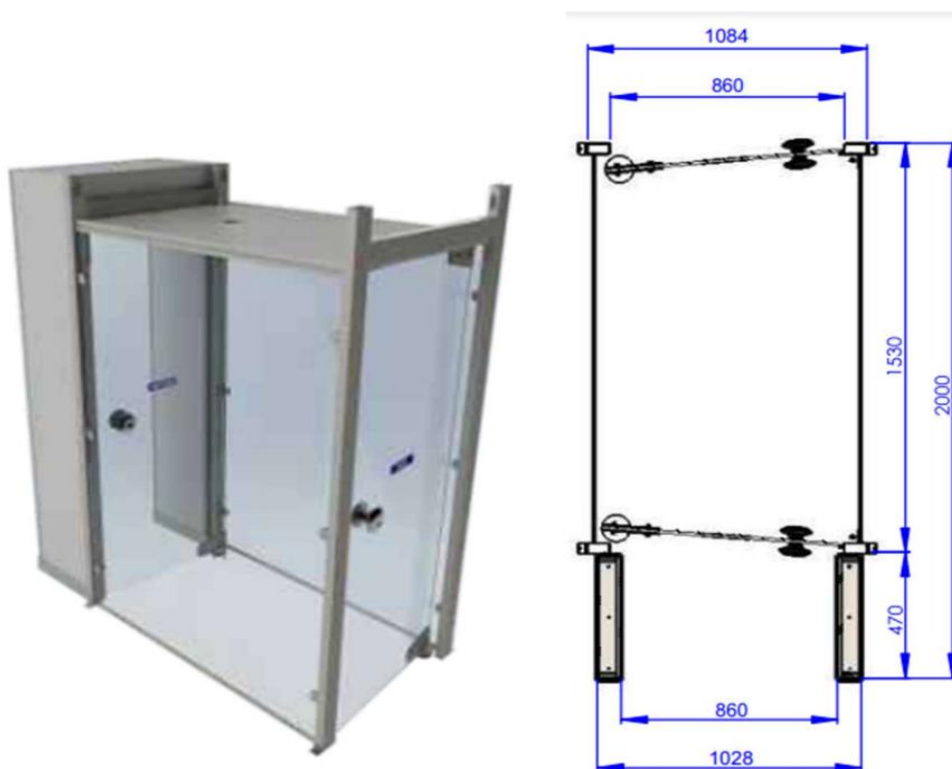
Imagem 04: PEDM modelos 1, 2, da tabela 03 acima.
