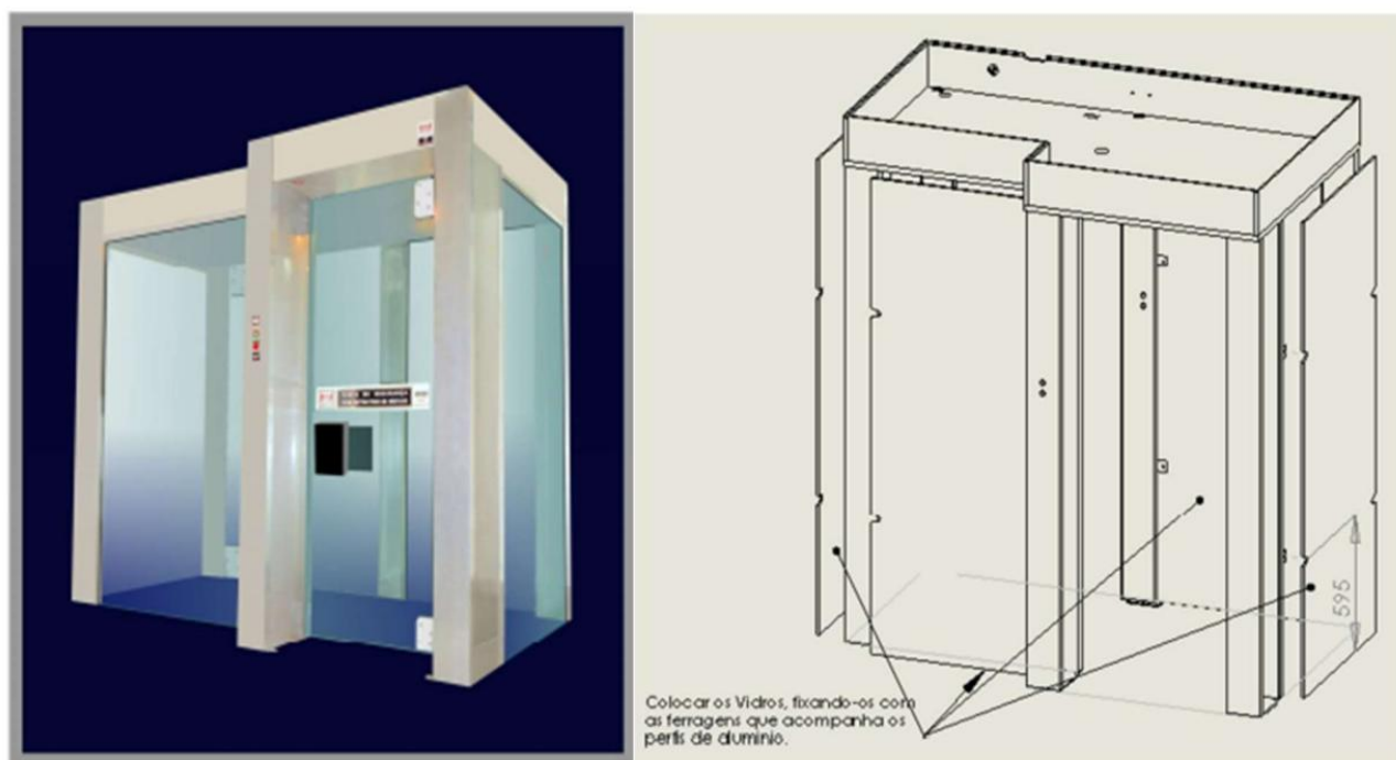
Imagem 02: Porta Eclusa Modelos 4 e 5 da tabela 01 acima.
