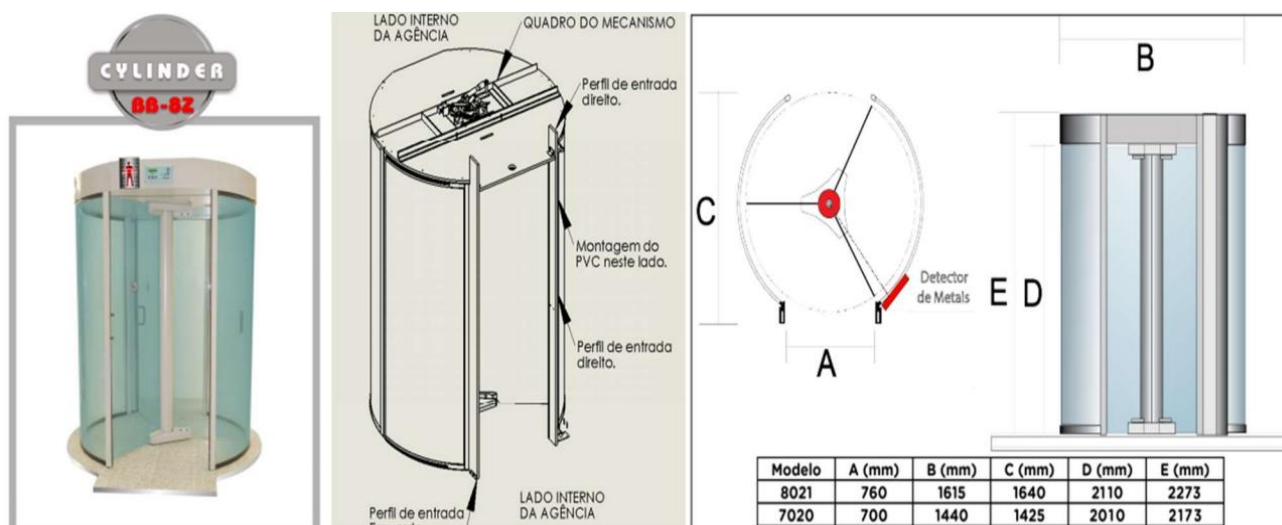
Imagem 01: Porta Giratória nos modelos 1,2,3 da tabela 01 acima.
