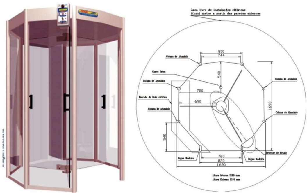
Imagem 03: PGDM modelos 1 e 3 da tabela 02 acima.
