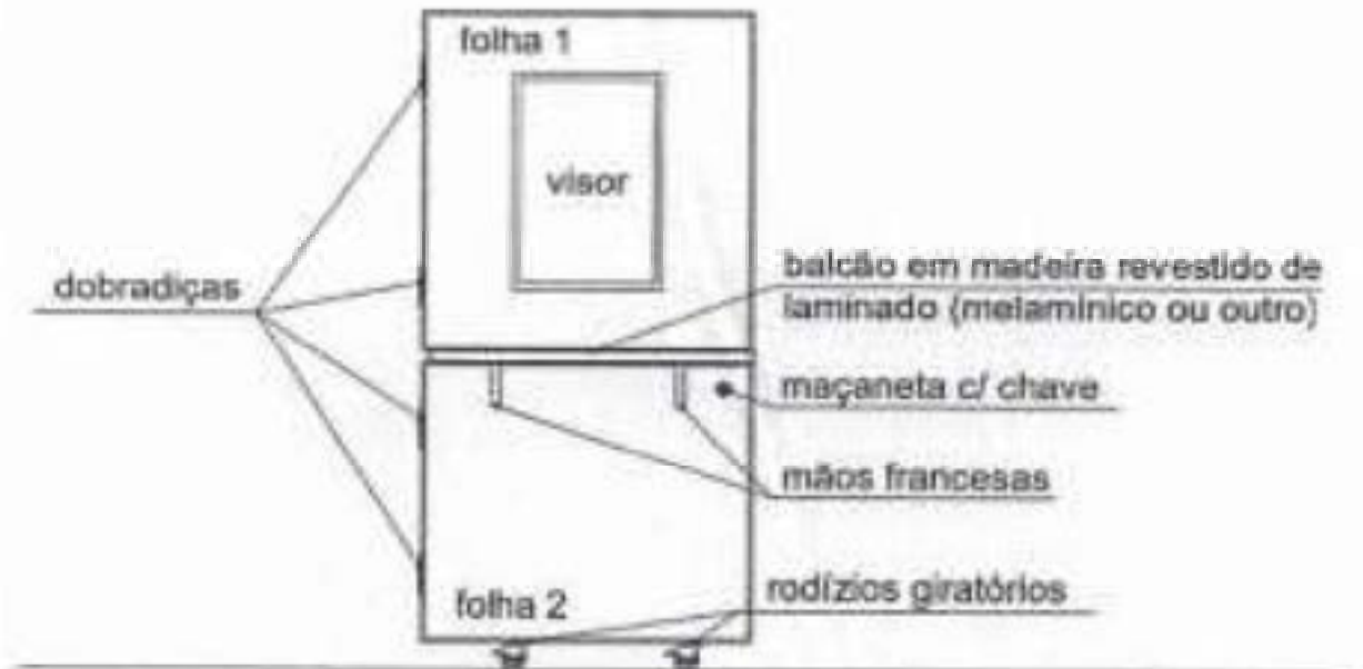
Porta balcão com duas folhas a/ esc.
