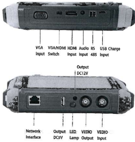
Figura 01: Monitor Testador CCTV AHD 1080P
