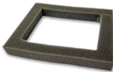
Exemplo de Calço de Espuma T-20 CALÇO DE ESPUMA VAZADO(220X170X30X20 MM) DENSIDADE 30KG/M3
